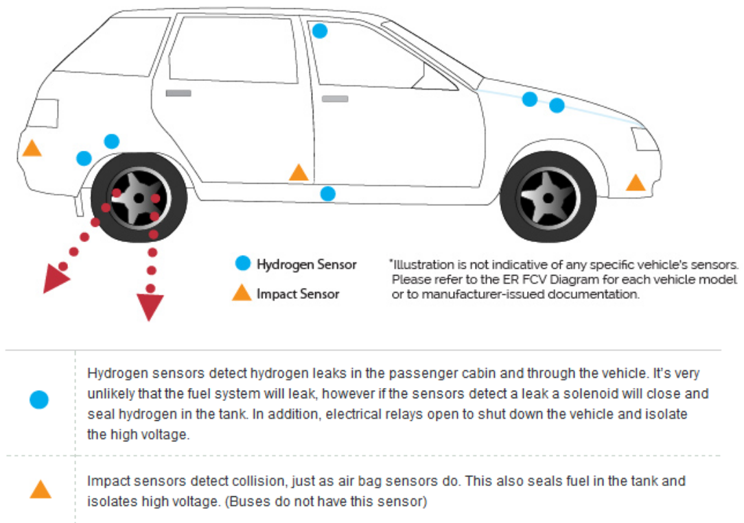
Abbildung 6. Mögliche Anordnung der Wasserstoffsensoren in einem FCEV [10].
