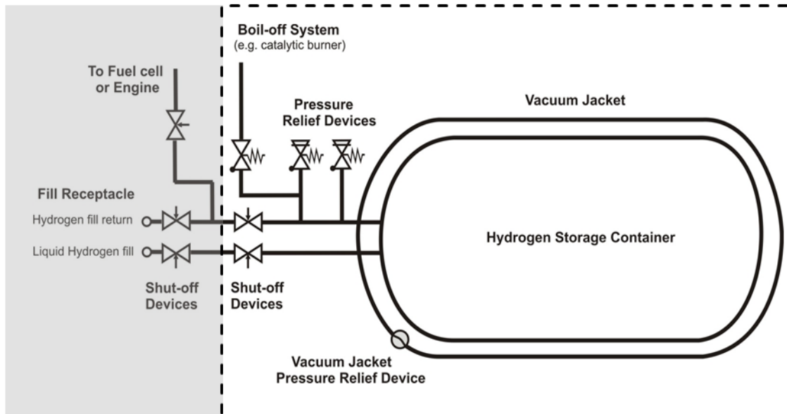
Abbildung 2. Eine schematische Darstellung des LH 2 -Speichersystems aus Ref. [8]
