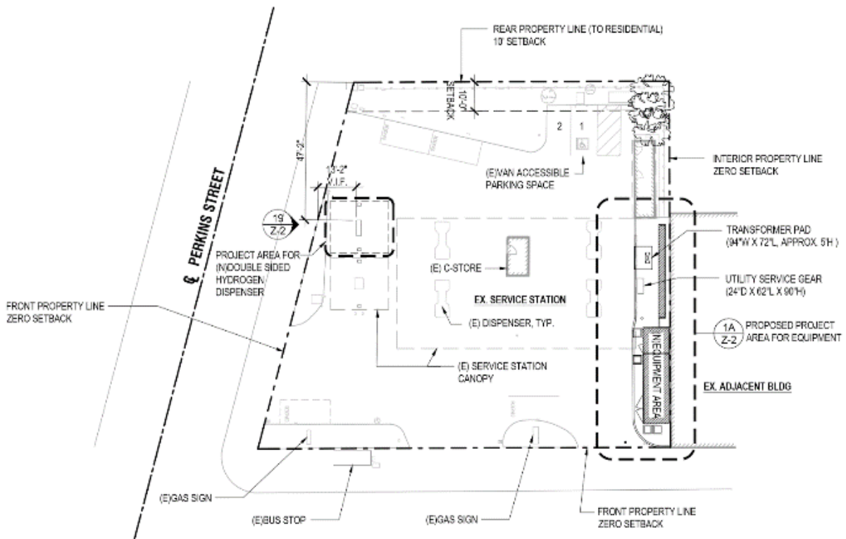
Abbildung 7. Linde LHRS und Anlage in Oakland. (Quellen: Linde)
