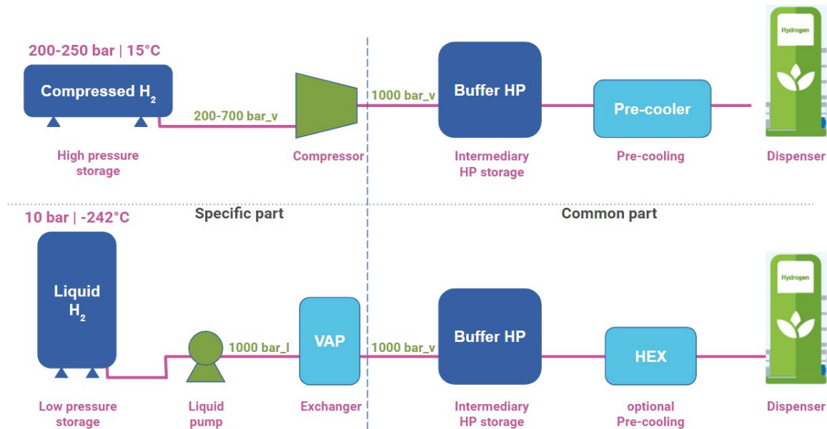
Abbildung 6. Vereinfachter Vergleich zwischen Tankstellen für gasförmigen und flüssigen Wasserstoff. Oben: gasförmiges HRS, unten flüssiges HRS.
