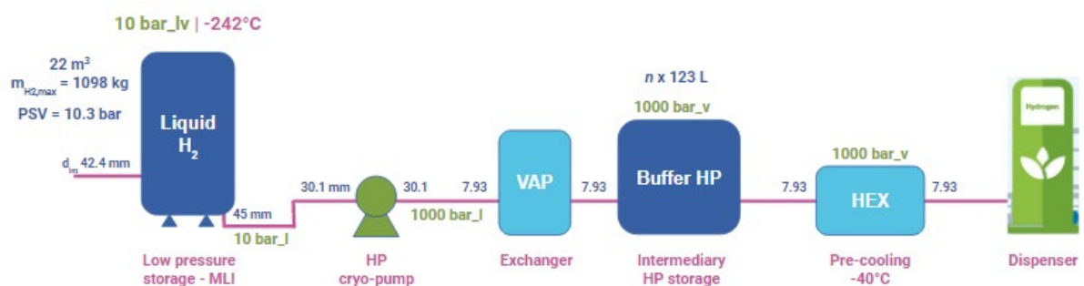
Abbildung 5. Vereinfachte Skizze einer Flüssigwasserstoff-Tankstelle.
