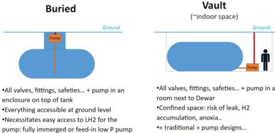
Abbildung 4. Die beiden wichtigsten möglichen Konzepte für unterirdische LH 2 -Speicher.
