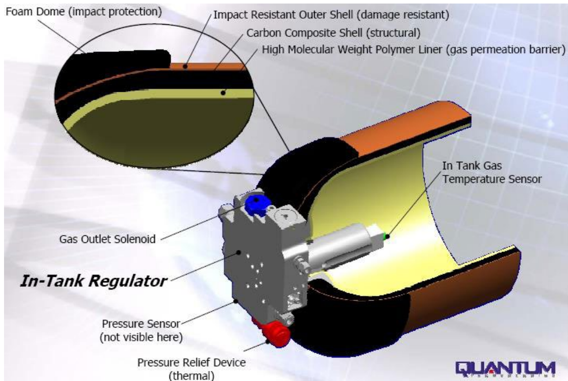
Obrázek 5. Průřez stěnou vodíkové nádrže Quantum s integrovanými systémy pro skladování paliva
